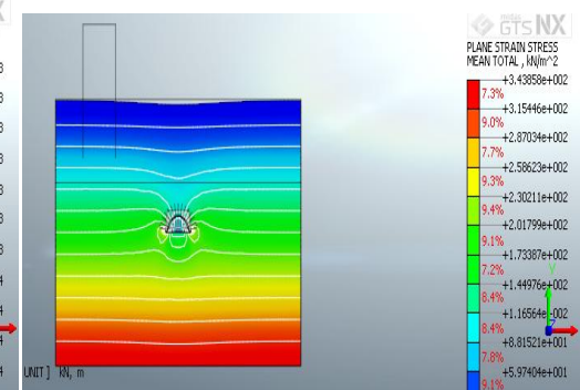
Fig 7 : Stress
